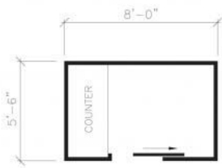
Sliding Door Left
